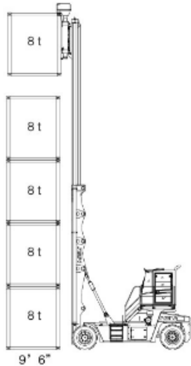
CPCD180EC5-CZ
