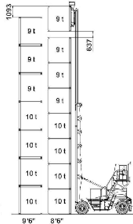
CPCD250EC8-VZG2
