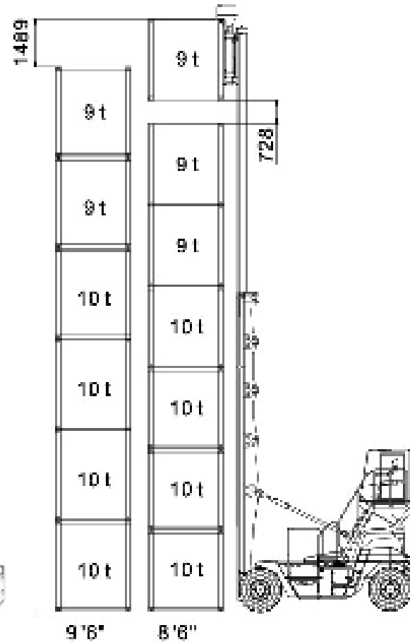
CPCD250EC7-VZG2
